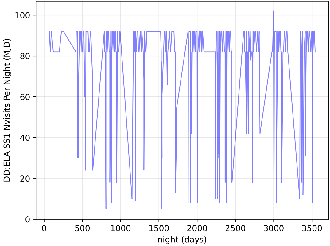
too_elab_r16_d3_ugrizy_v3.4_10yrs all bands: DD:ELAISS1 Nvisits Per Night
