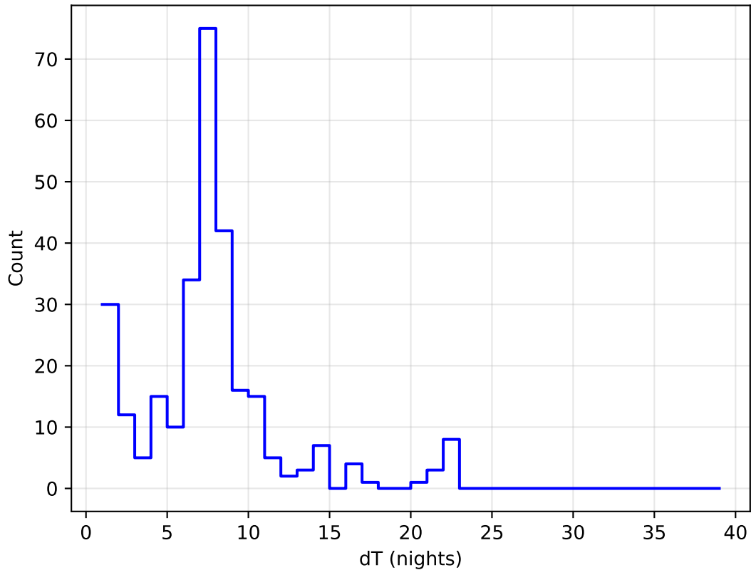
too_elab_r16_d3_ugrizy_v3.4_10yrs all bands: DD:EDFS Delta Nights Histogram
