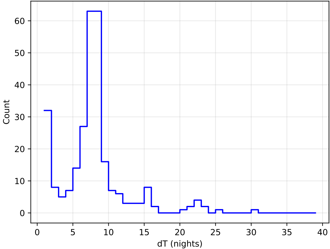
too_elab_r16_d3_ugrizy_v3.4_10yrs all bands: DD:ECDFS Delta Nights Histogram
