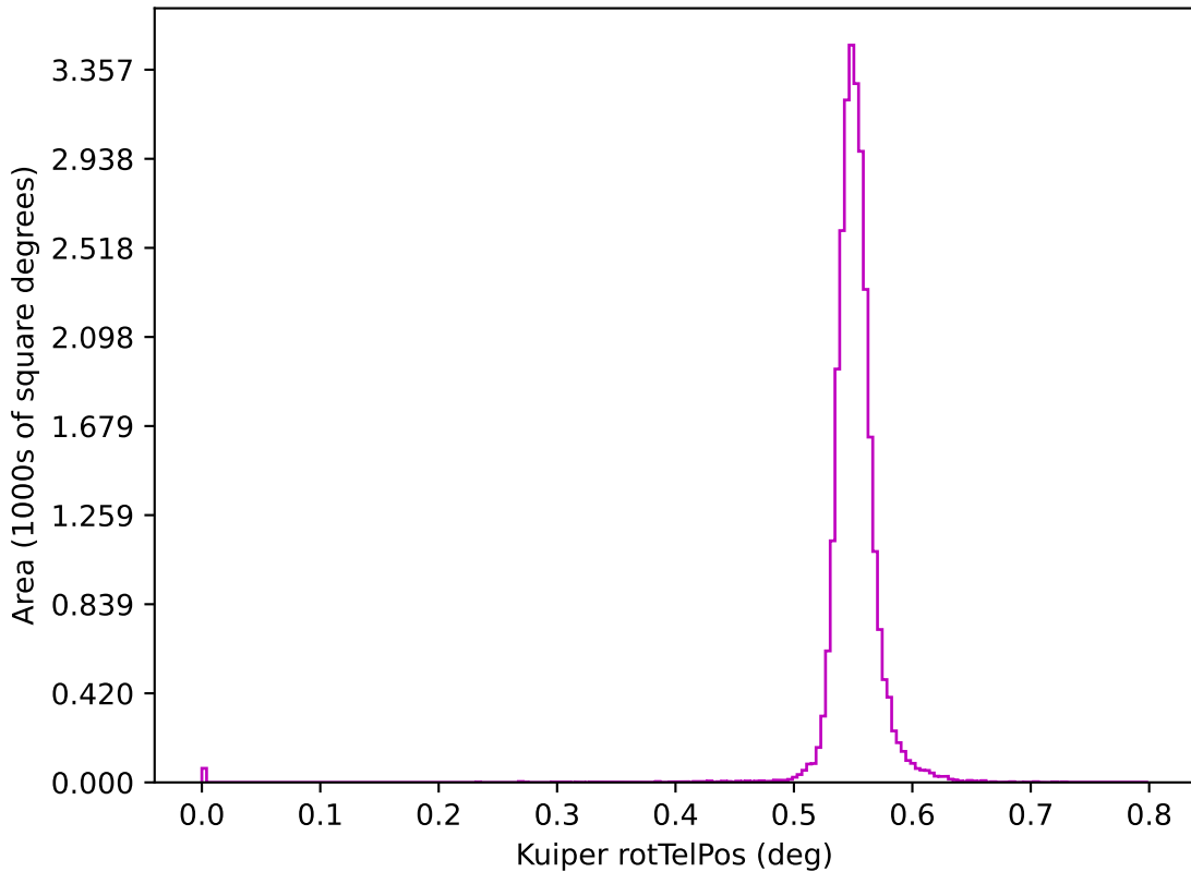
too_elab_r16_d3_gz_v3.4_10yrs z: Kuiper rotTelPos
