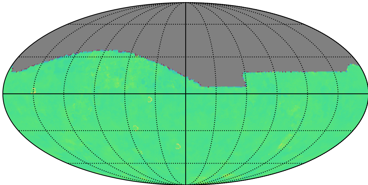
too_elab_r16_d3_griz_v3.4_10yrs z: Kuiper rotTelPos
