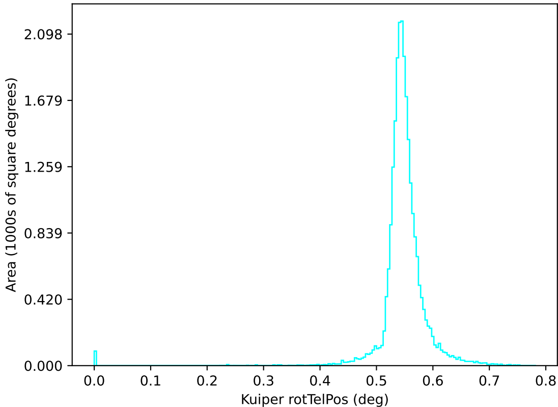
too_elab_r16_d3_griz_v3.4_10yrs u: Kuiper rotTelPos
