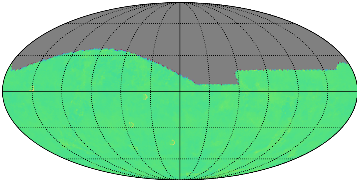
too_elab_r16_d3_griz_v3.4_10yrs i: Kuiper rotTelPos
