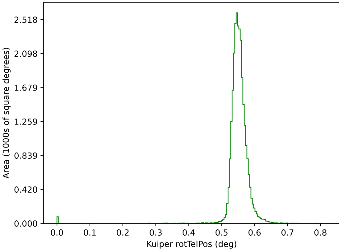
too_elab_r16_d3_griz_v3.4_10yrs g: Kuiper rotTelPos
