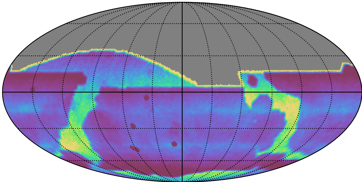
too_elab_r16_d3_griz_v3.4_10yrs : DCRprecision
