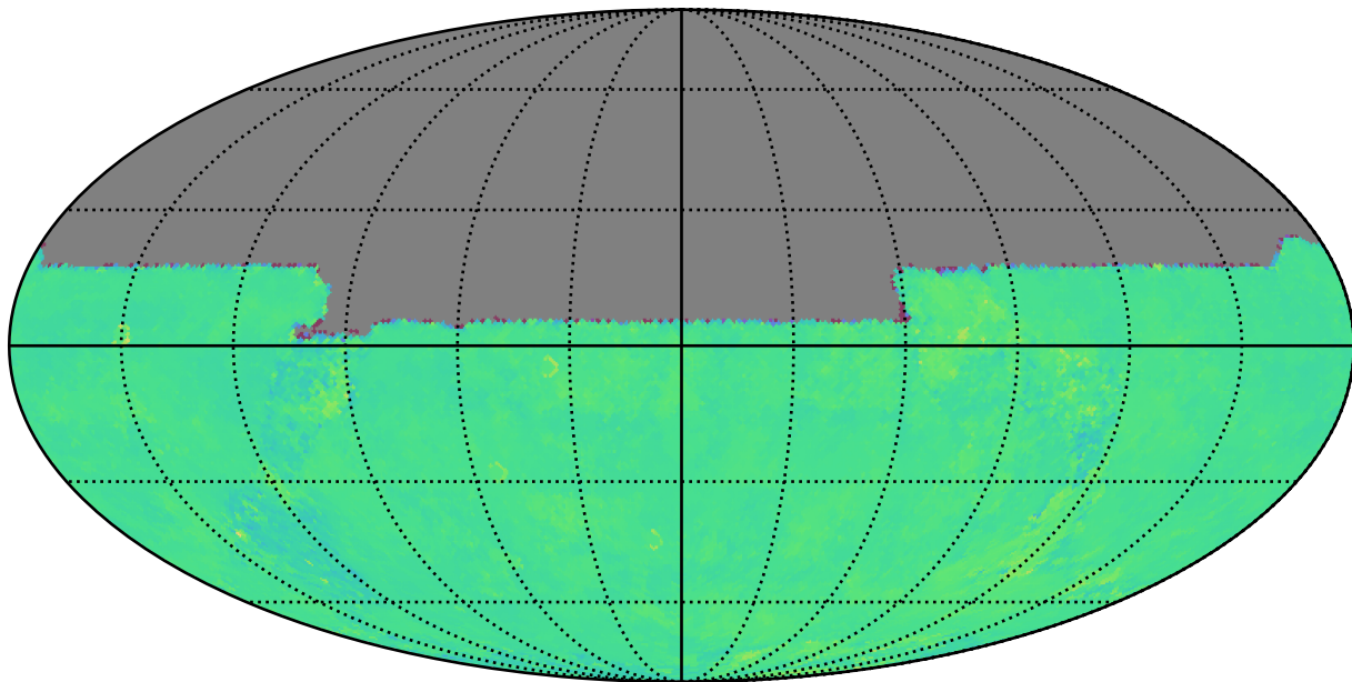
too_elab_r16_d3_giz_v3.4_10yrs u: Kuiper rotTelPos
