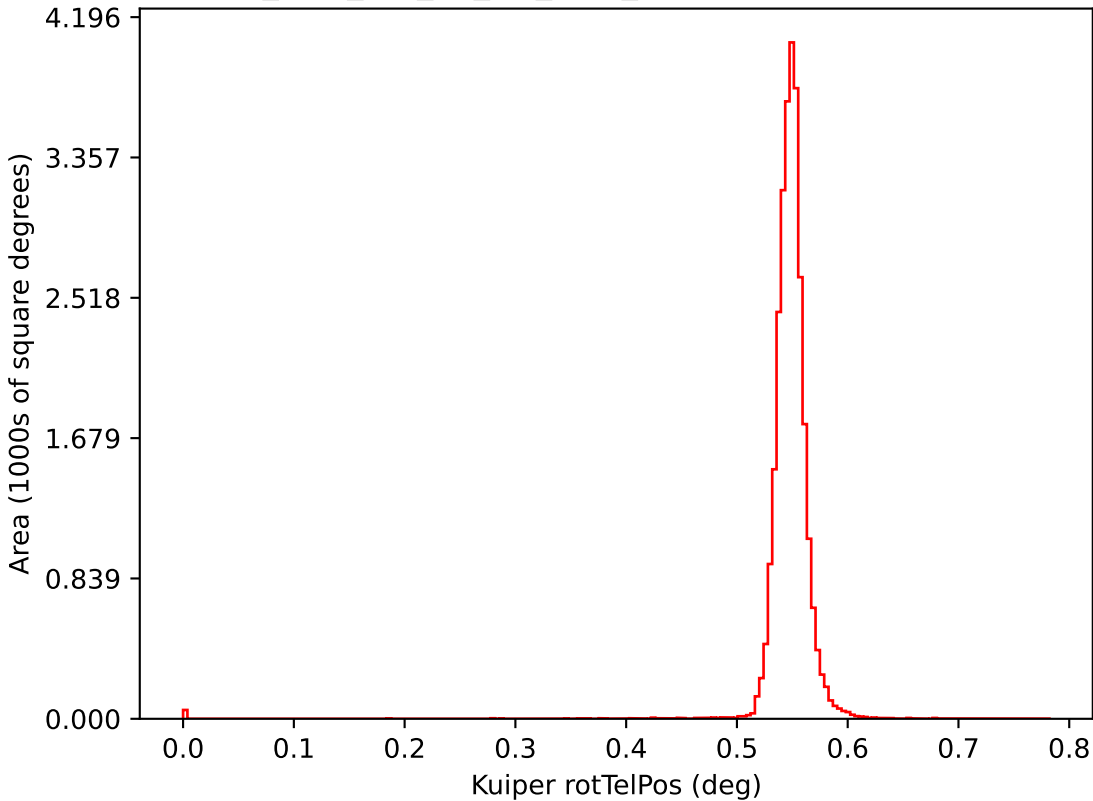
too_elab_r16_d3_giz_v3.4_10yrs i: Kuiper rotTelPos
