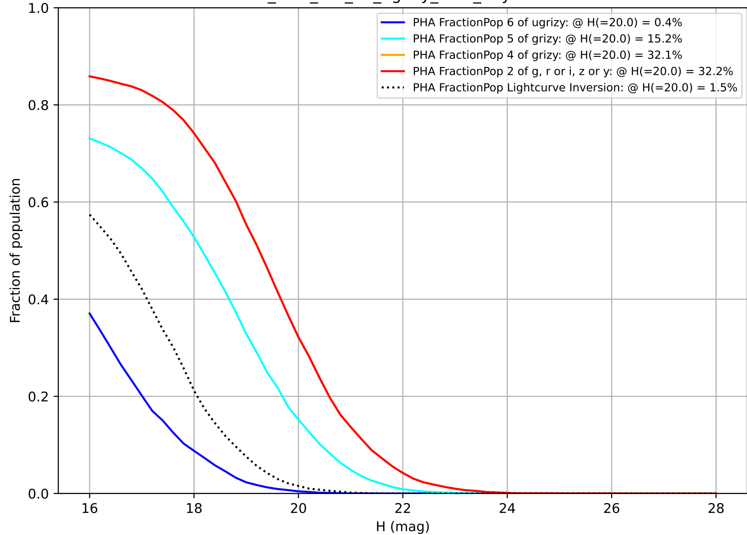
too_elab_r16_d2_ugrizy_v3.4_10yrs PHA
