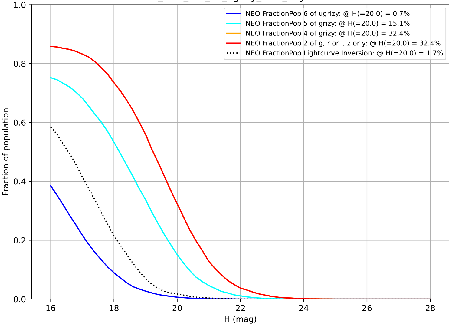
too_elab_r16_d2_ugrizy_v3.4_10yrs NEO
