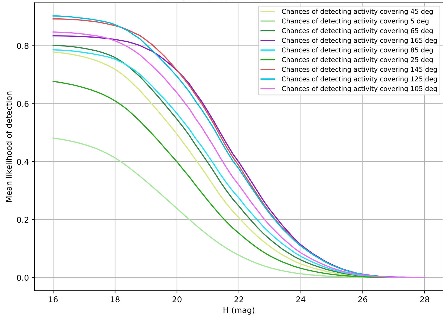
too_elab_r16_d2_ugrizy_v3.4_10yrs NEO
