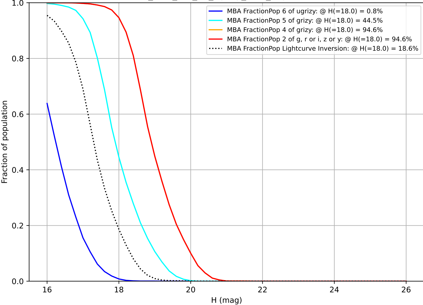
too_elab_r16_d2_ugrizy_v3.4_10yrs MBA
