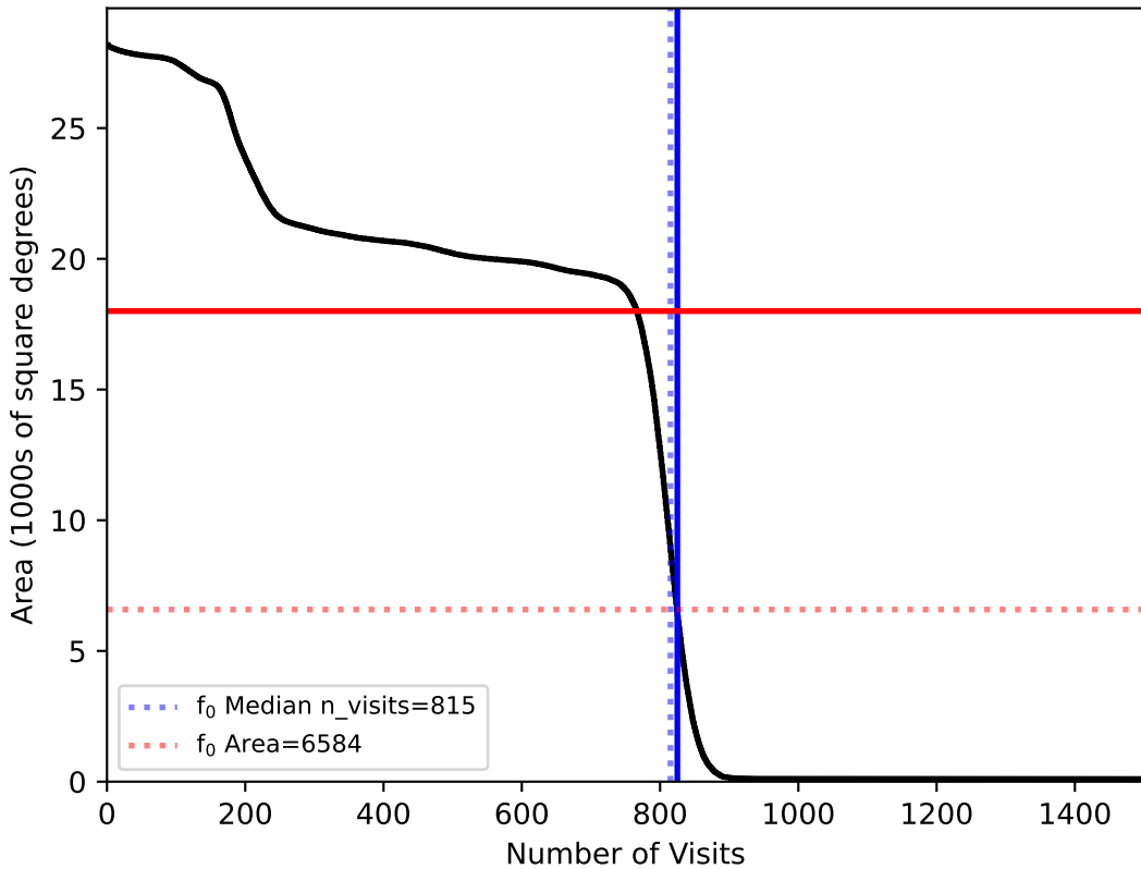
too_elab_r16_d2_ugrizy_v3.4_10yrs : f0
