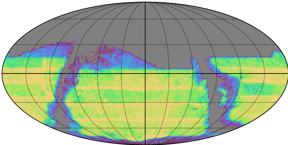
too_elab_r16_d2_ugrizy_v3.4_10yrs : TDC_rate
