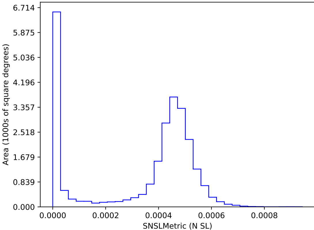
too_elab_r16_d2_ugrizy_v3.4_10yrs : SNSLMetric
