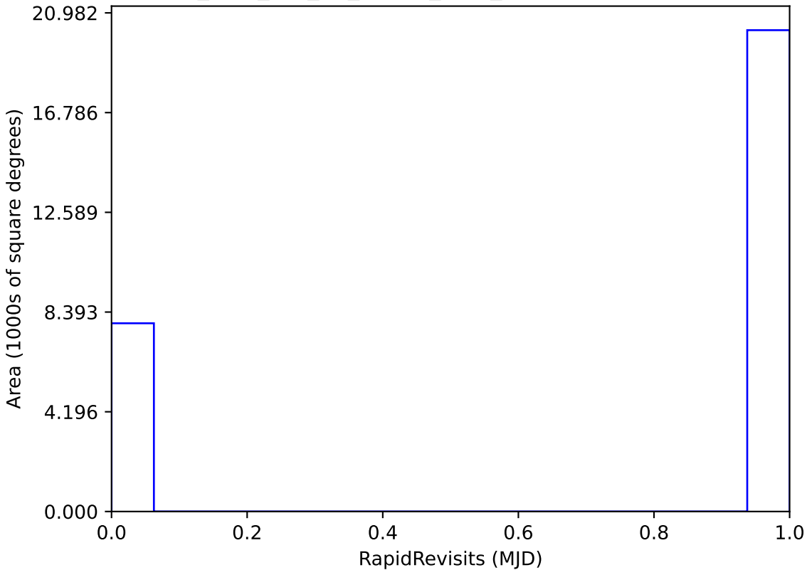
too_elab_r16_d2_ugrizy_v3.4_10yrs : RapidRevisits
