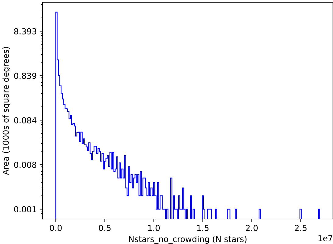
too_elab_r16_d2_ugrizy_v3.4_10yrs i: Nstars_no_crowding
