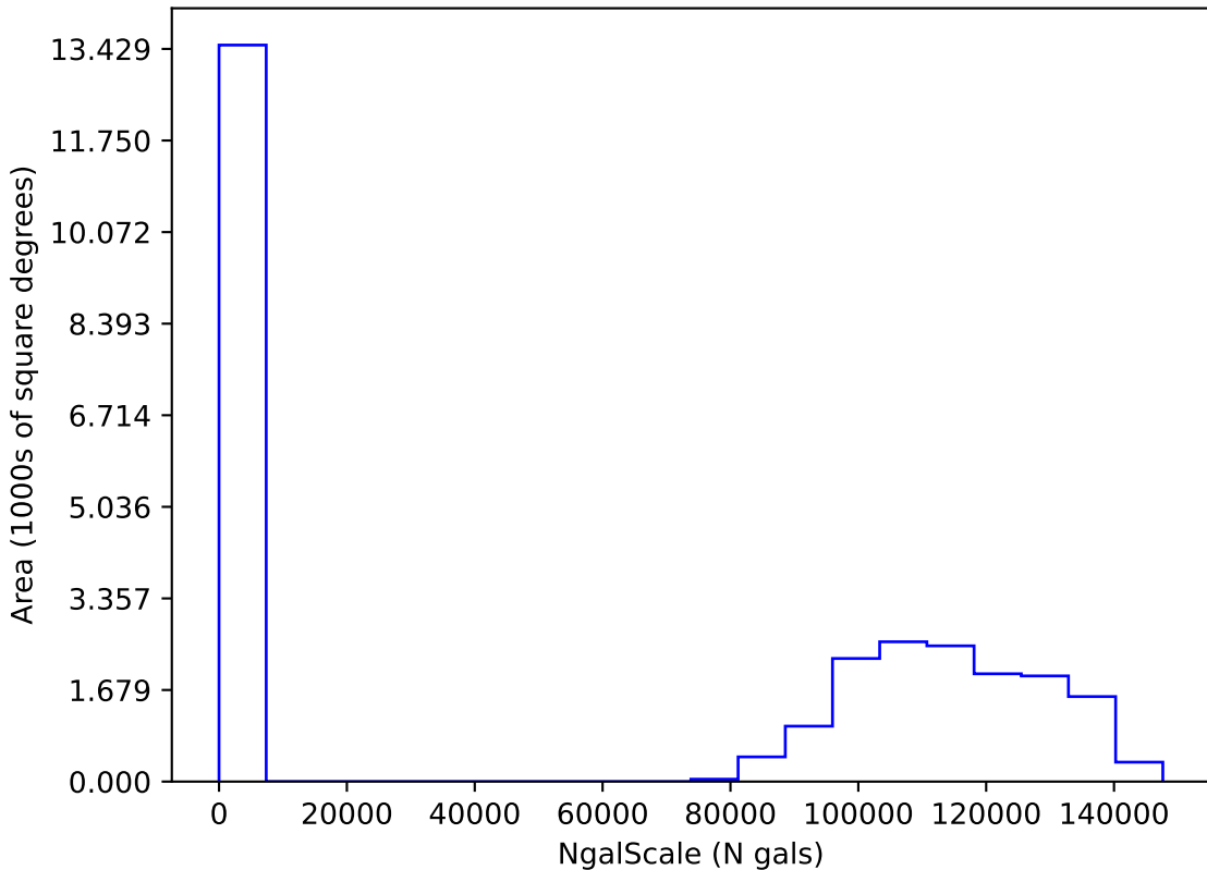
too_elab_r16_d2_ugrizy_v3.4_10yrs i: NgalScale
