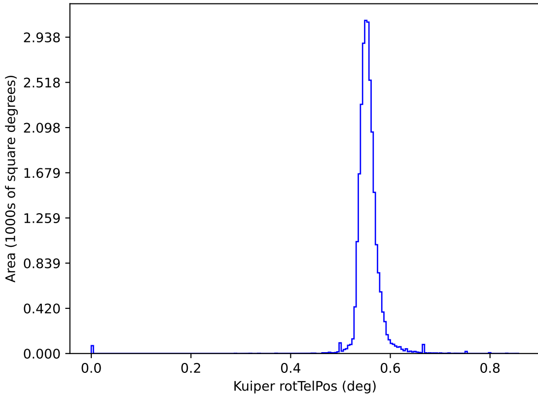
too_elab_r16_d2_ugrizy_v3.4_10yrs y: Kuiper rotTelPos
