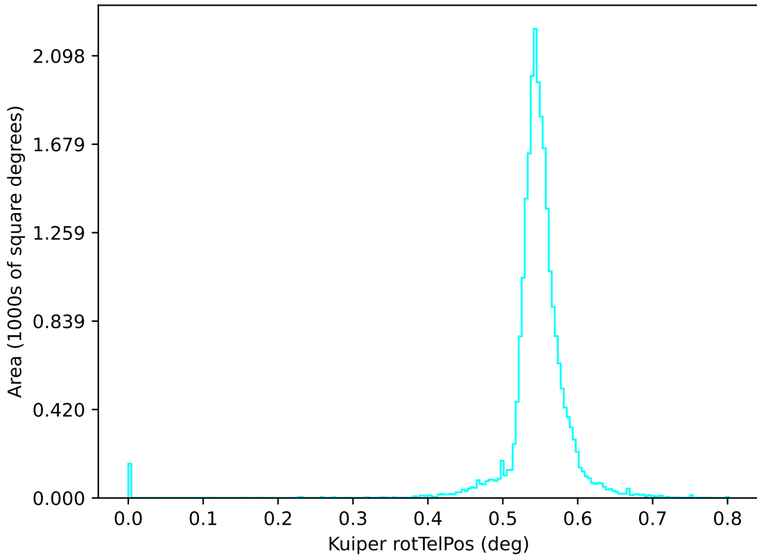
too_elab_r16_d2_ugrizy_v3.4_10yrs u: Kuiper rotTelPos
