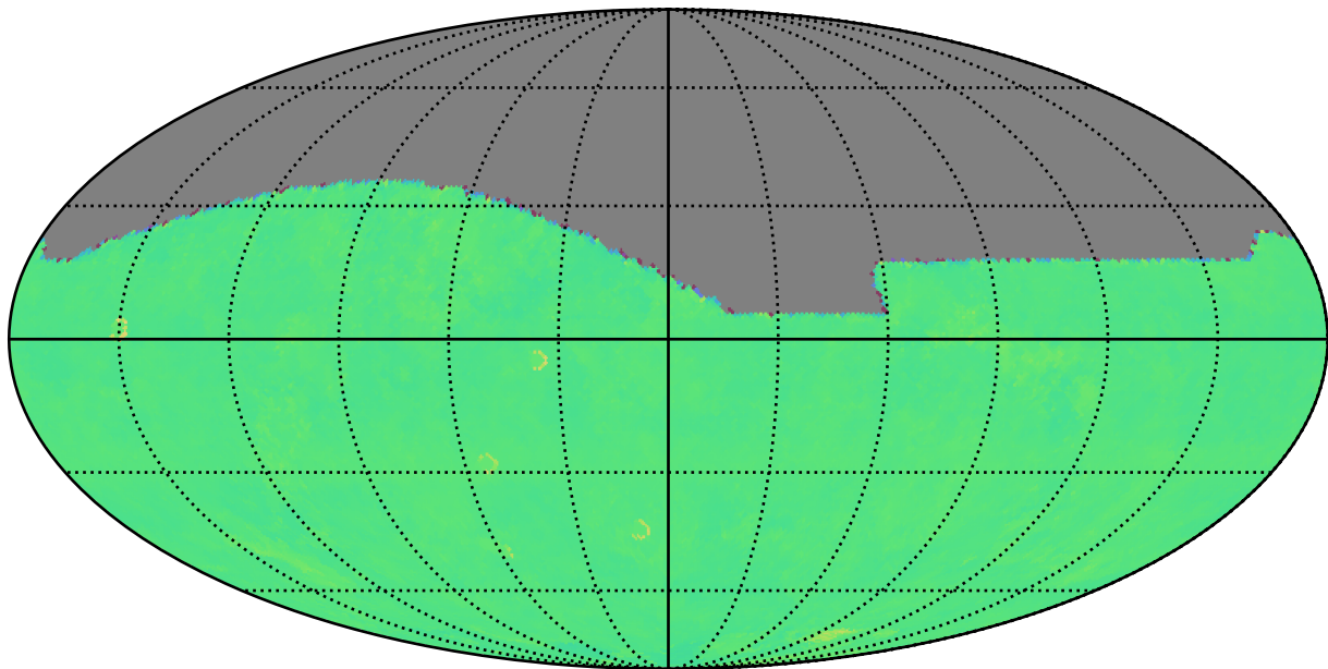
too_elab_r16_d2_ugrizy_v3.4_10yrs i: Kuiper rotTelPos
