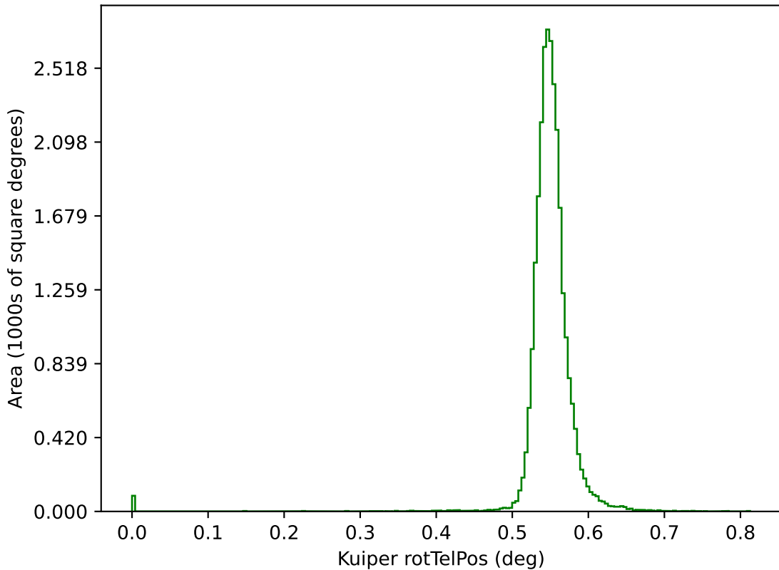
too_elab_r16_d2_ugrizy_v3.4_10yrs g: Kuiper rotTelPos
