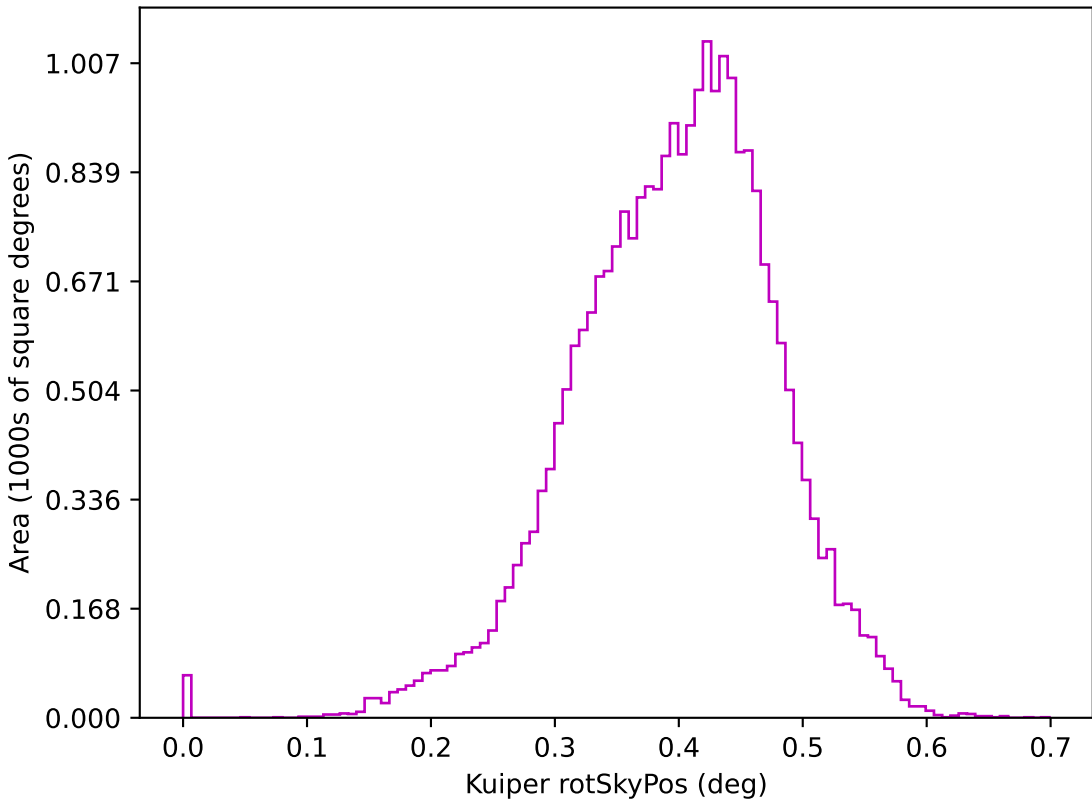
too_elab_r16_d2_ugrizy_v3.4_10yrs z: Kuiper rotSkyPos
