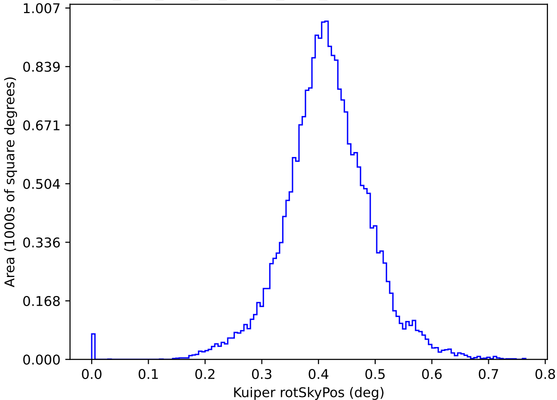
too_elab_r16_d2_ugrizy_v3.4_10yrs y: Kuiper rotSkyPos
