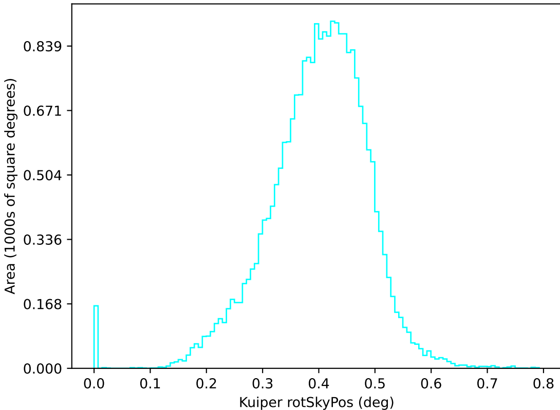
too_elab_r16_d2_ugrizy_v3.4_10yrs u: Kuiper rotSkyPos
