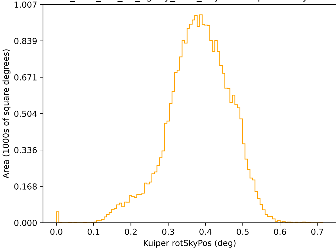
too_elab_r16_d2_ugrizy_v3.4_10yrs r: Kuiper rotSkyPos
