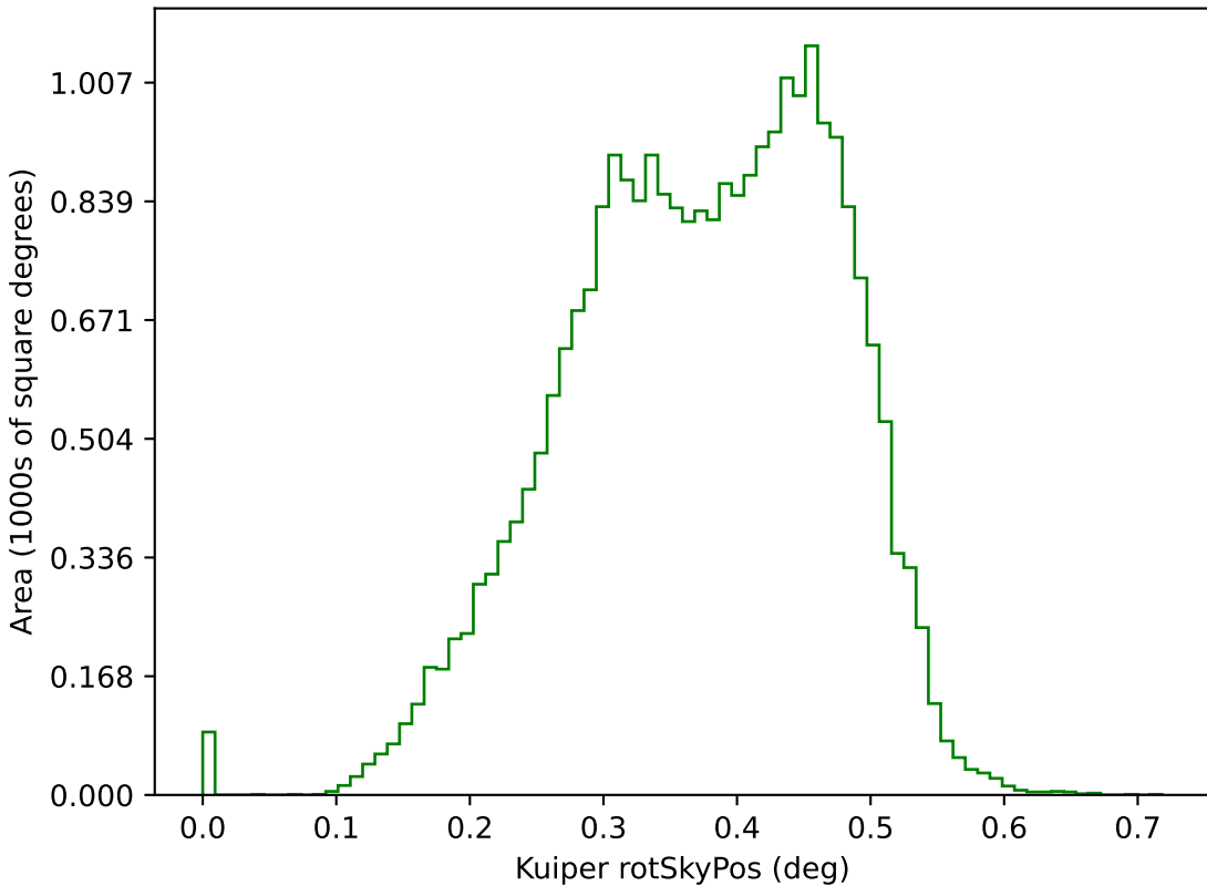
too_elab_r16_d2_ugrizy_v3.4_10yrs g: Kuiper rotSkyPos
