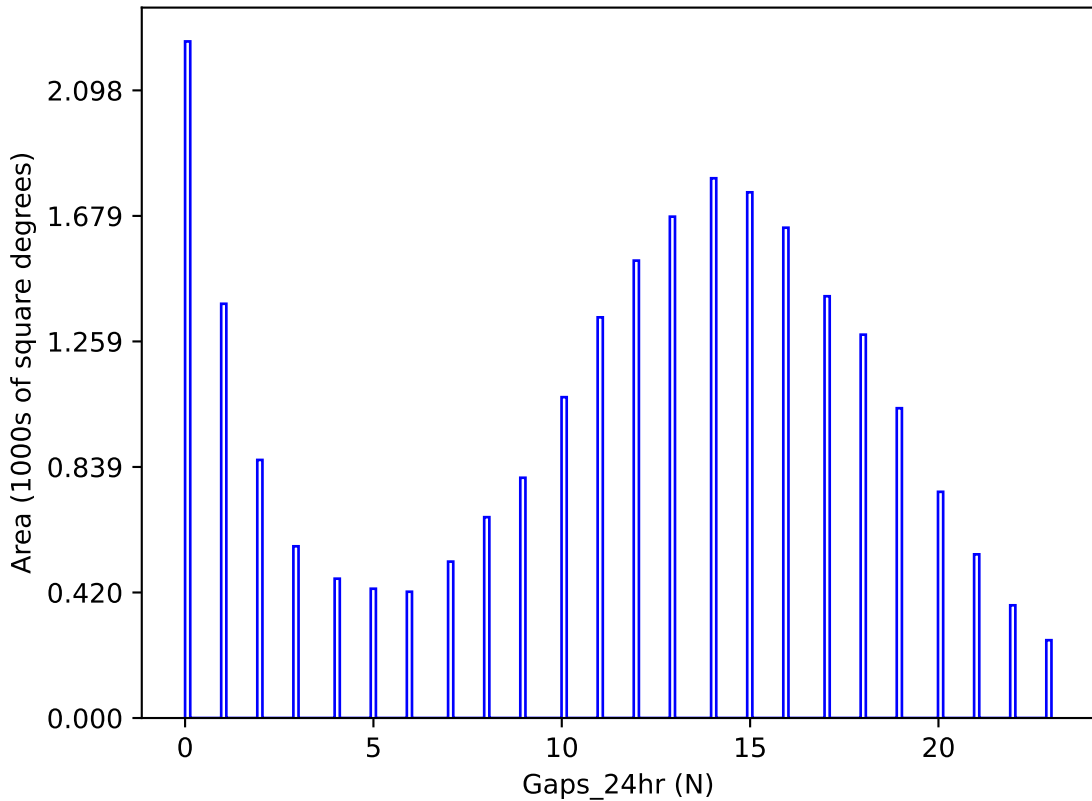
too_elab_r16_d2_ugrizy_v3.4_10yrs y band: Gaps_24hr
