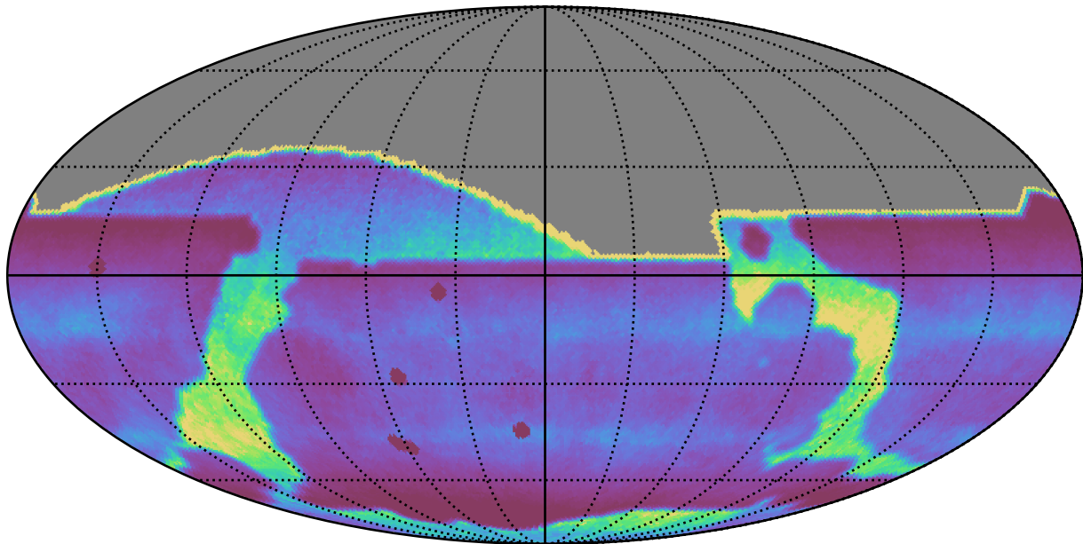
too_elab_r16_d2_ugrizy_v3.4_10yrs : DCRprecision
