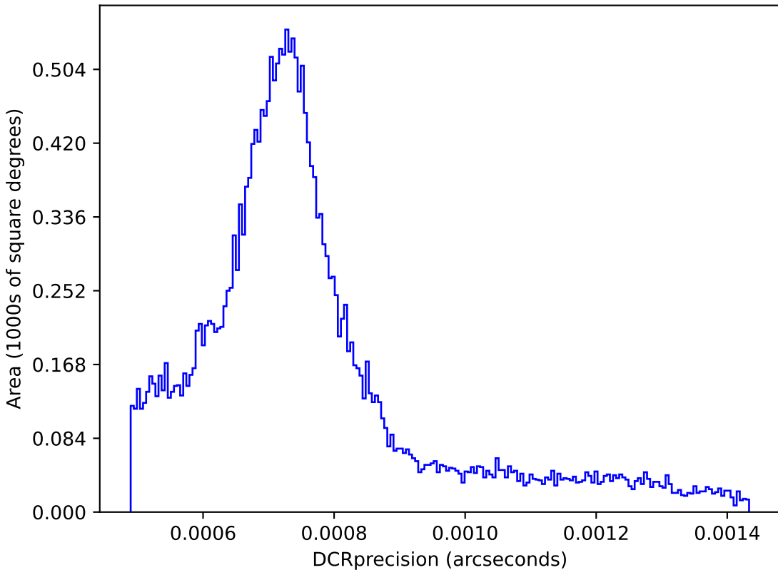
too_elab_r16_d2_ugrizy_v3.4_10yrs : DCRprecision
