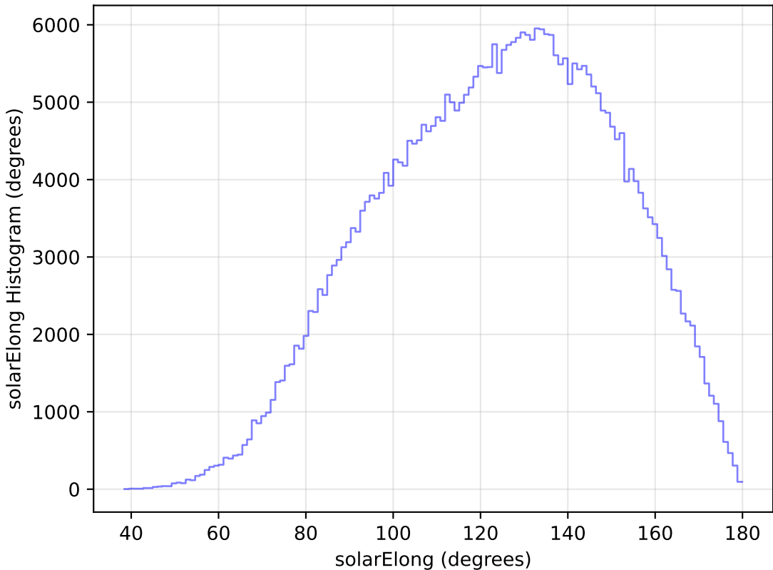
too_elab_r16_d2_ugrizy_v3.4_10yrs WFD y band: solarElong Histogram
