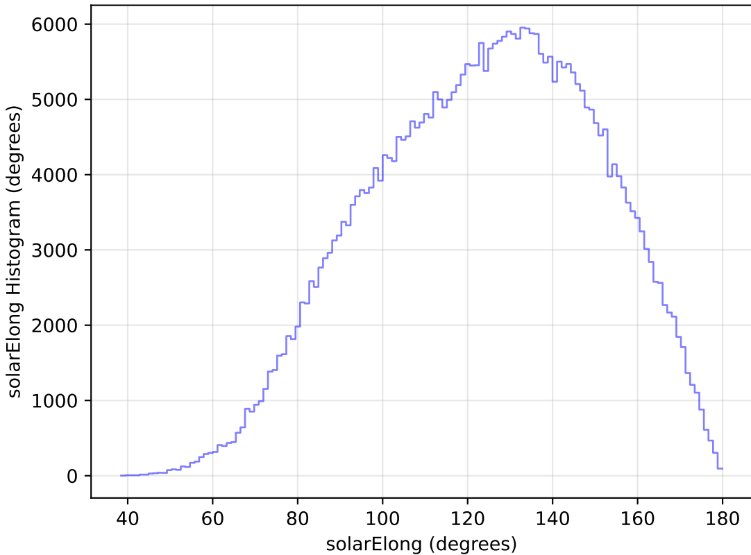
too_elab_r16_d2_ugrizy_v3.4_10yrs All sky y band: solarElong Histogram
