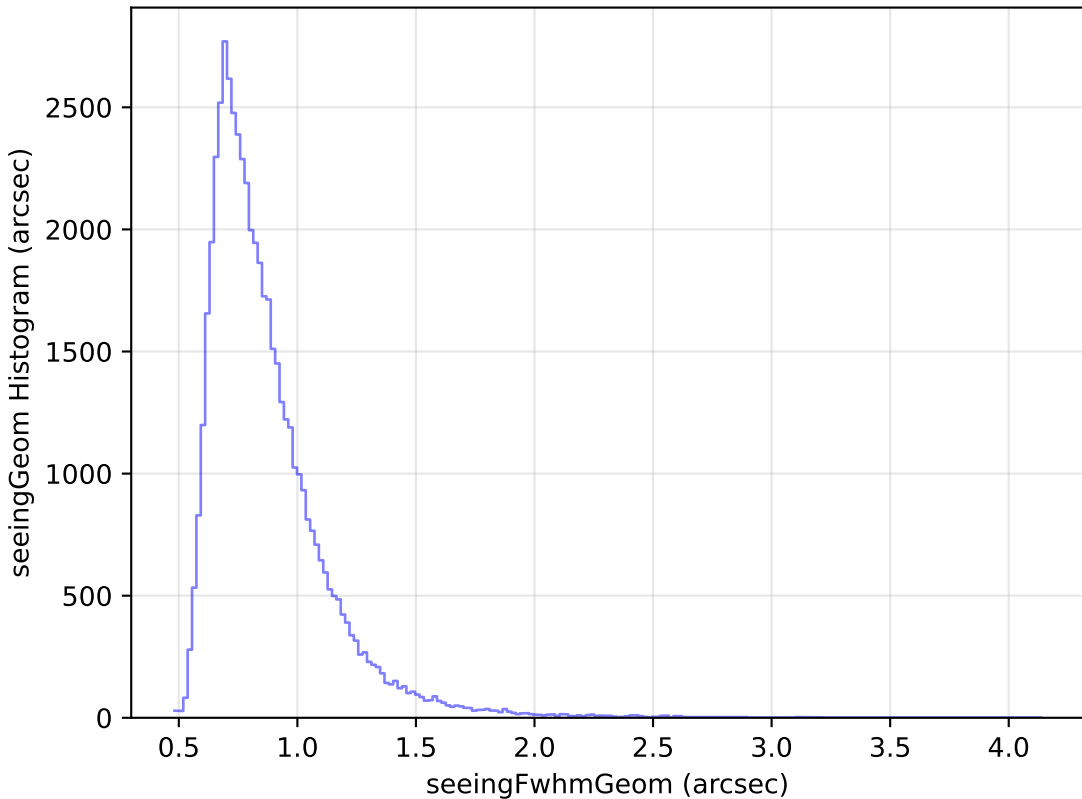
too_elab_r16_d2_ugrizy_v3.4_10yrs Yr 1 i band: seeingGeom Histogram
