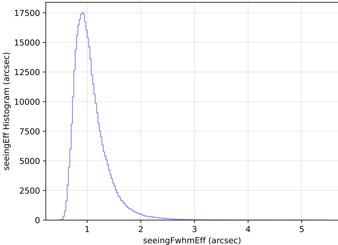
too_elab_r16_d2_ugrizy_v3.4_10yrs WFD y band: seeingEff Histogram
