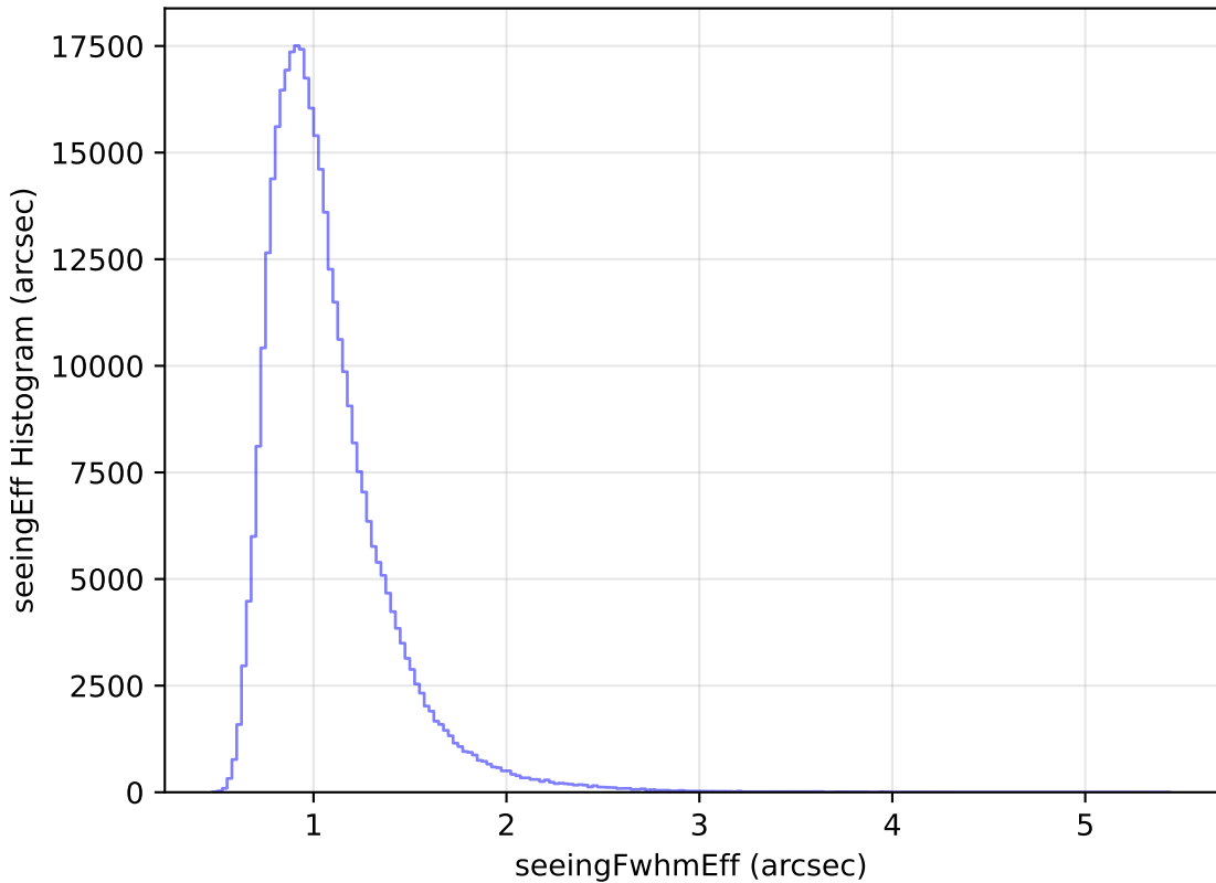
too_elab_r16_d2_ugrizy_v3.4_10yrs All sky y band: seeingEff Histogram
