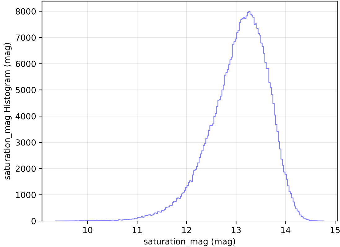
too_elab_r16_d2_ugrizy_v3.4_10yrs WFD y band: saturation_mag Histogram
