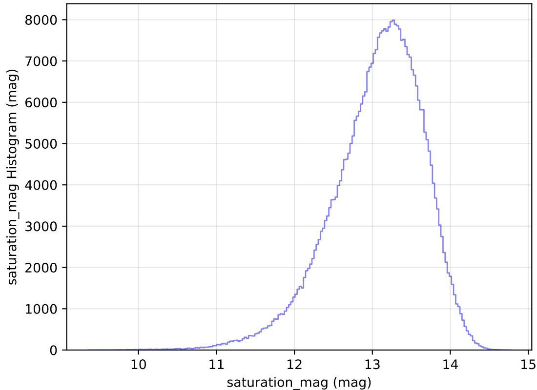
too_elab_r16_d2_ugrizy_v3.4_10yrs All sky y band: saturation_mag Histogram
