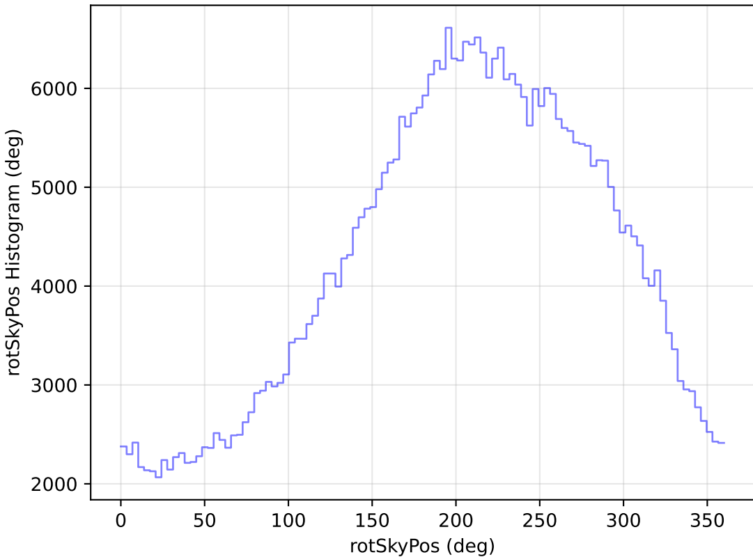
too_elab_r16_d2_ugrizy_v3.4_10yrs WFD z band: rotSkyPos Histogram
