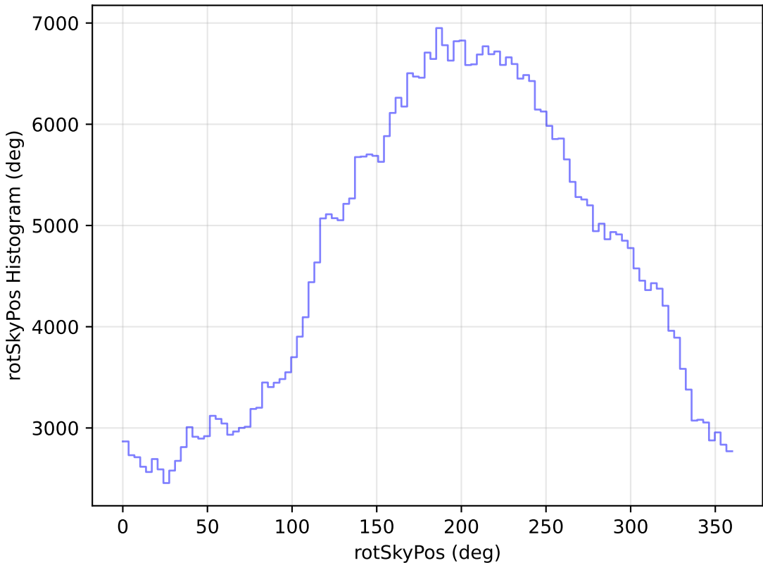
too_elab_r16_d2_ugrizy_v3.4_10yrs WFD r band: rotSkyPos Histogram
