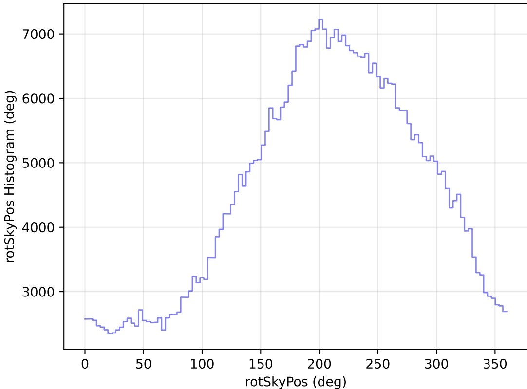
too_elab_r16_d2_ugrizy_v3.4_10yrs WFD i band: rotSkyPos Histogram
