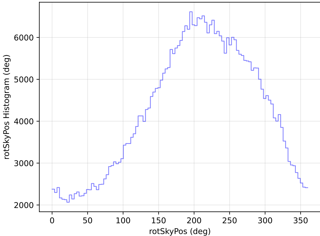
too_elab_r16_d2_ugrizy_v3.4_10yrs All sky z band: rotSkyPos Histogram
