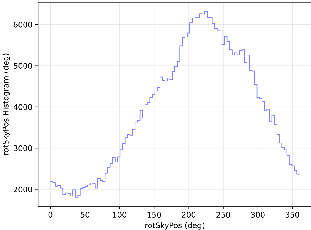
too_elab_r16_d2_ugrizy_v3.4_10yrs All sky y band: rotSkyPos Histogram
