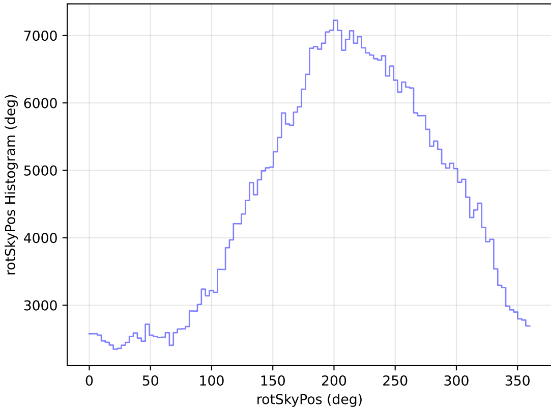
too_elab_r16_d2_ugrizy_v3.4_10yrs All sky i band: rotSkyPos Histogram
