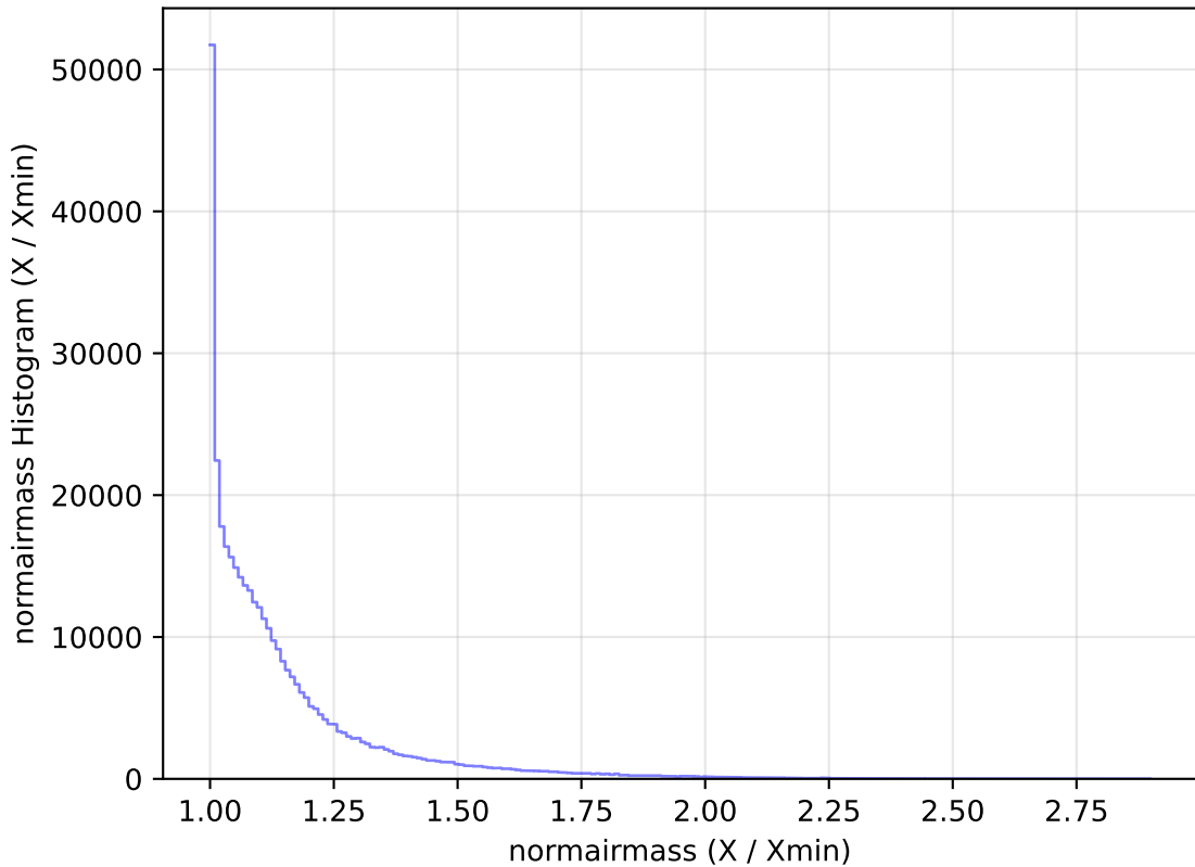
too_elab_r16_d2_ugrizy_v3.4_10yrs All sky y band: normairmass Histogram
