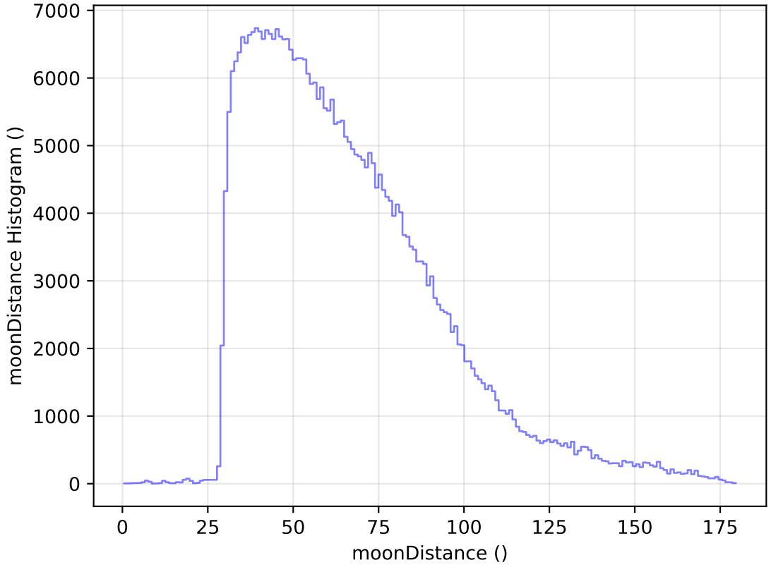
too_elab_r16_d2_ugrizy_v3.4_10yrs WFD y band: moonDistance Histogram
