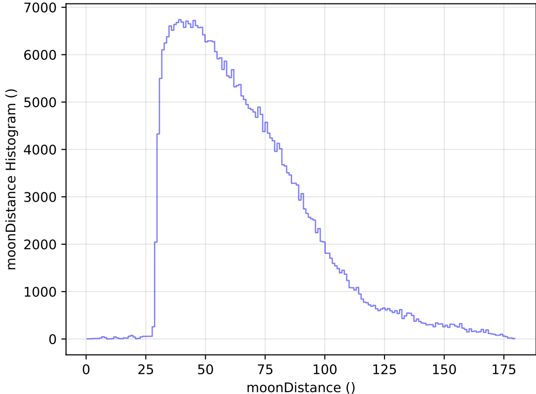
too_elab_r16_d2_ugrizy_v3.4_10yrs All sky y band: moonDistance Histogram
