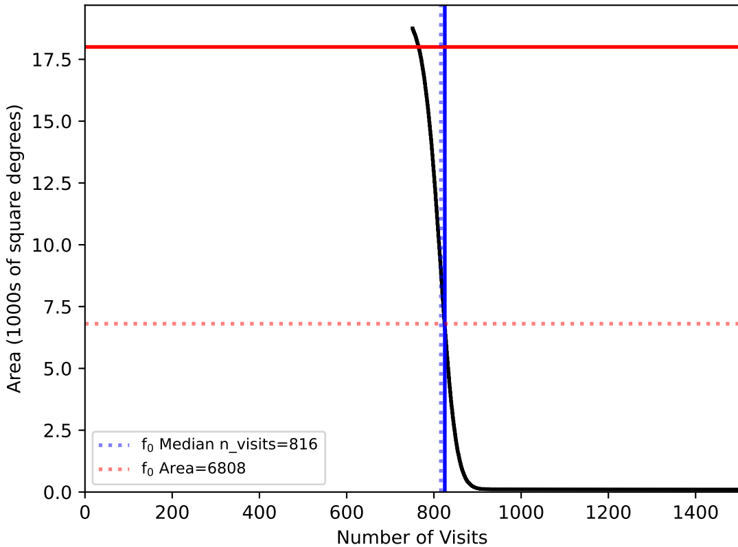
too_elab_r16_d2_ugrizy_v3.4_10yrs WFD: f0
